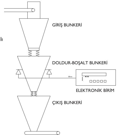
Şekil 9: Doldur-Boşalt Kantarı Şematik Gösterim
