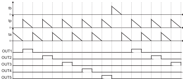
Şekil 4.1: nGrP = 1, noLt = 5 iken çalışma diyagramı
