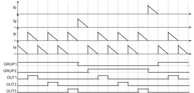
Şekil 4.2: nGrP = 2, noLt = 3 ve tL P = tL P1 iken çalışma diyagramı
