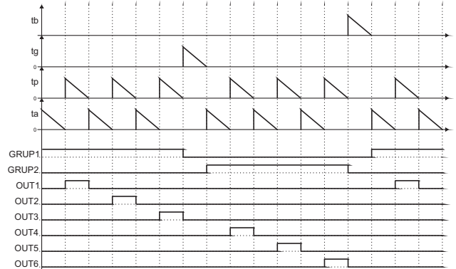
Şekil 4.3: nGrP = 2, noLt = 3 ve tL P = tL P2 iken çalışma diyagramı
