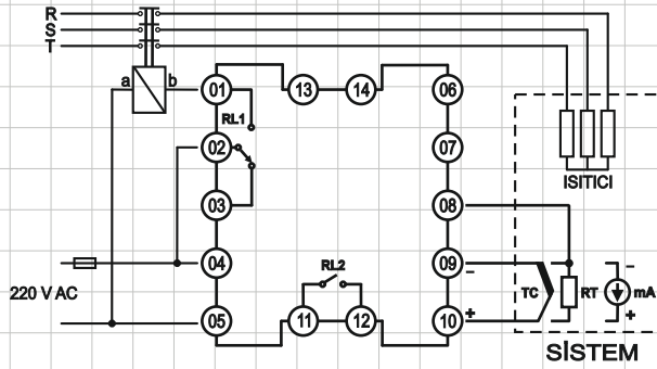
Şekil 6.1 E-50 Bağlantı Şeması
