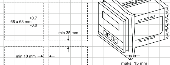
Şekil 5.2 Pano Kesiti ve Minimum Aralıklar
